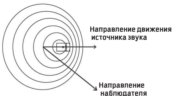
Рисунок 4. Эффект Доплера, когда направление движения источника звука и наблюдателя не совпадают
